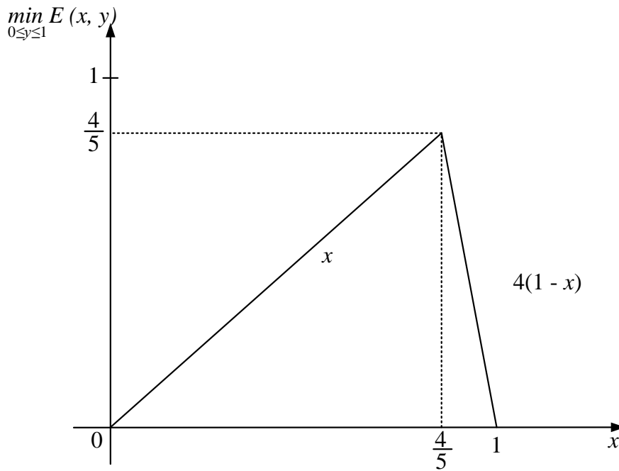
Рисунок 6.15 – Графік функції \min_{0 \leq y \leq 1} E(x, y)
