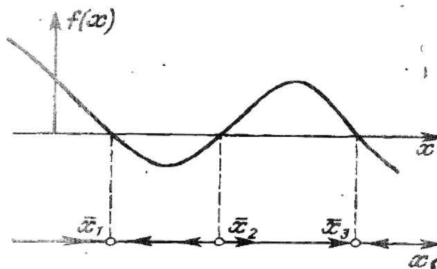
Фазова пряма
