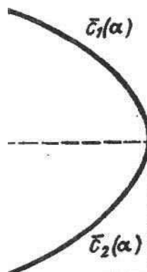
Рисунок 5.8 – Залежність стаціонарної концентрації клітин \bar{c} від параметра \alpha для рівняння (5.15)
