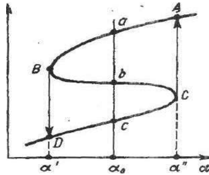
Рисунок 5.9 – Залежність правої частини рівняння (5.15) від параметра \alpha
