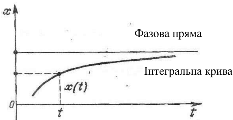
Рисунок 5.4 – Залежність змінної x від часу t для рівняння (5.7)
