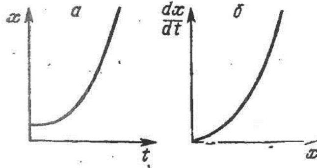
Рисунок 6.1 – Залежність чисельності популяції від часу (а) та швидкості зростання від чисельності (б) відповідно до формули (5.6)
