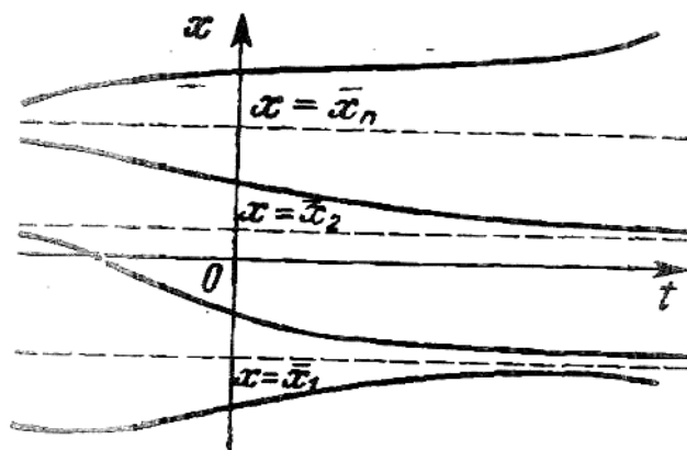
Рисунок 5.1 – Інтегральні криві t, x ; \bar{x}_1, \bar{x}_2, \dots, \bar{x}_n – розв'язки рівняння (5.7)
