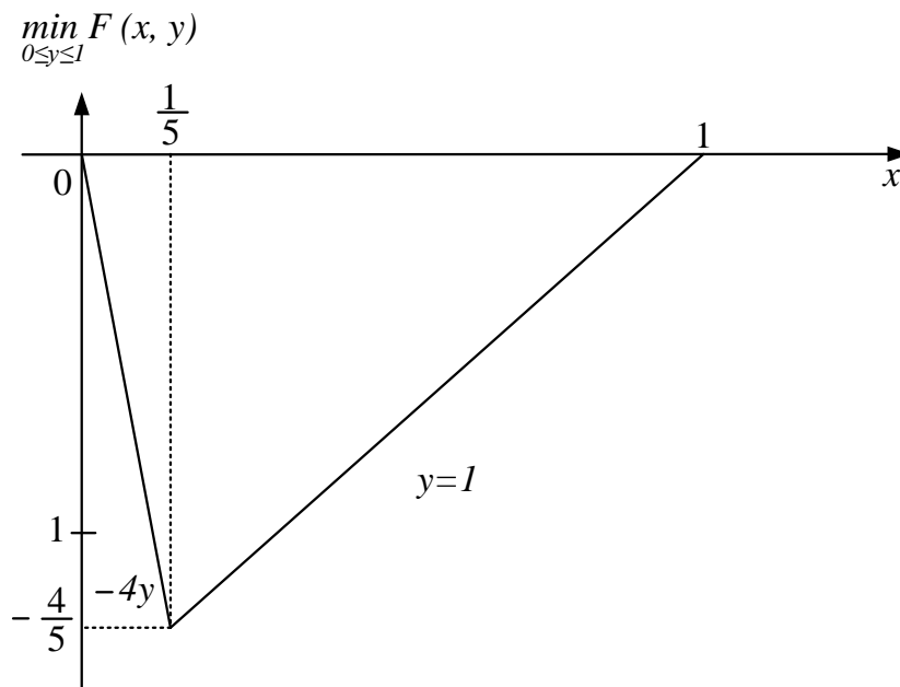
Рисунок 6.16 – Графік функції \min_{0 \leq y \leq 1} F(x, y)
