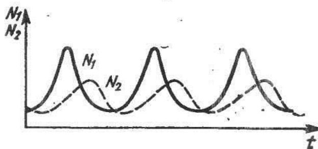
Рисунок 5.21 – Залежність чисельності хижаків N_2 і жертви N_1 від часу
