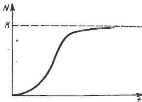
Рисунок 5.6 – Логістична крива
