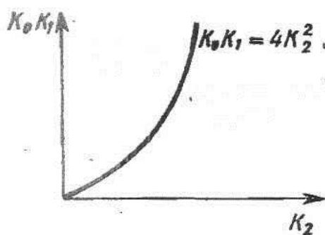
Рисунок 5.18 – Площина параметрів для системи рівнянь (5.49)
